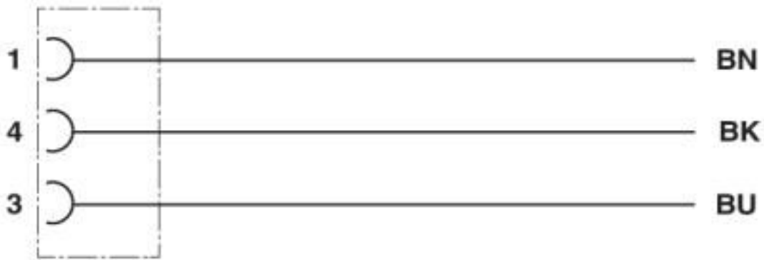
Diagrama eléctrico
