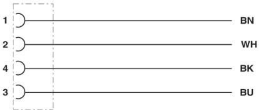
Diagrama eléctrico
