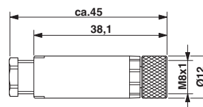
Esquema de dimensiones
