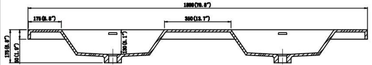
SECTION A-A
