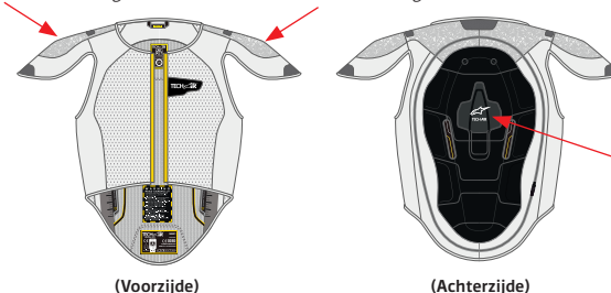
(Voorzijde) (Achterzijde) Afbeelding 1 – Locaties sensoren
