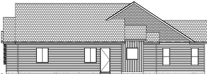
RIGHT ELEVATION
