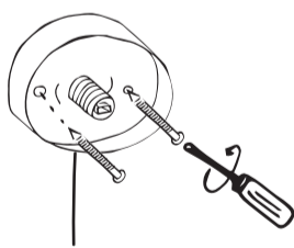
7 Vissez le col sur le support
