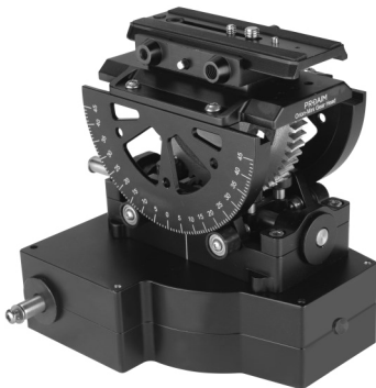
Orion Mini Geared Head
