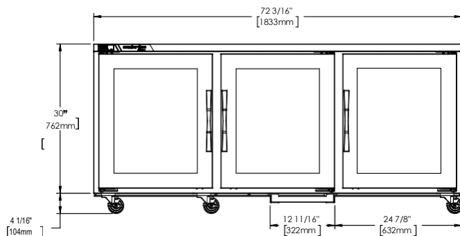
ELEVACIÓN
