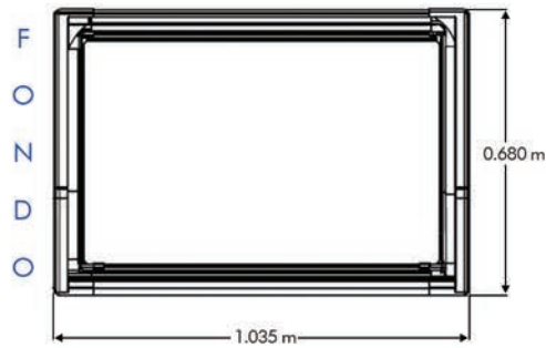
• VISTA TOP
