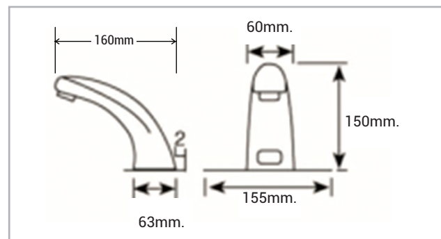
MEDIDAS DE LA LLAVE
