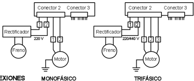
FIG. A2 CONEXIONES MONOFÁSICO
