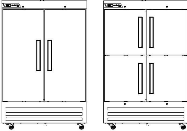
ELEVACIÓN
