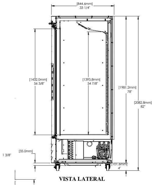
ELEVACIÓN
