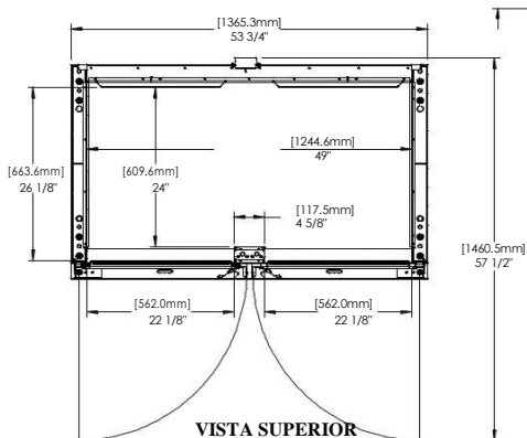
VISTA SUPERIOR
