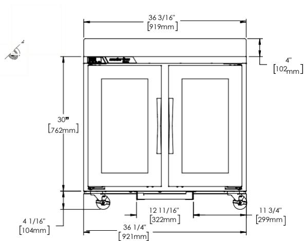
ELEVACIÓN
