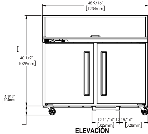
ELEVACION
