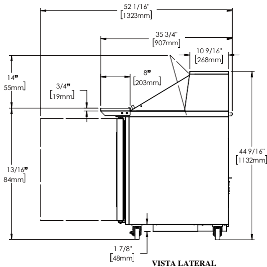
VISTA LATERAL
