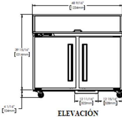
ELEVACIÓN
