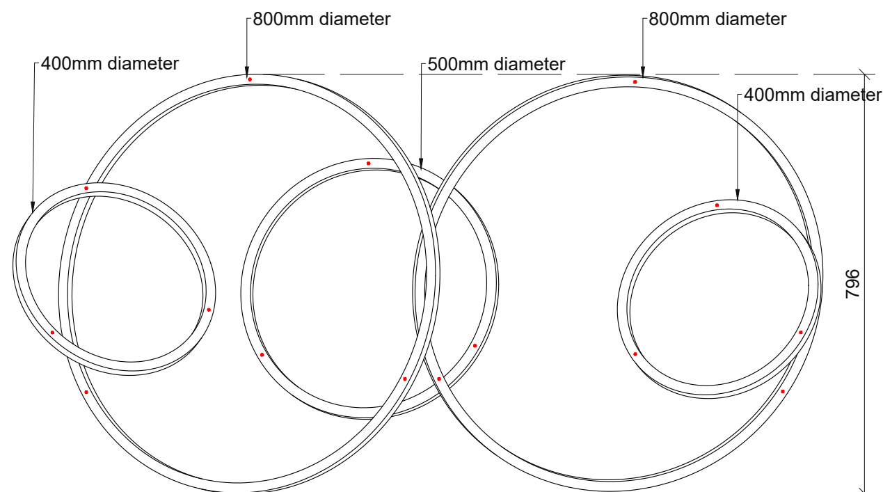
02-Ceiling Plan-Lohja Tornio
