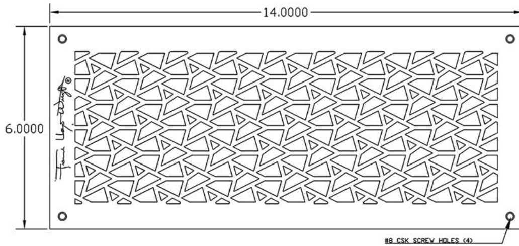
(A) PLAN SCALE: 6" = 1'
