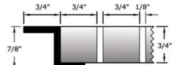
EC 300 C FRAME
