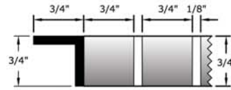
EC 300 B FRAME
