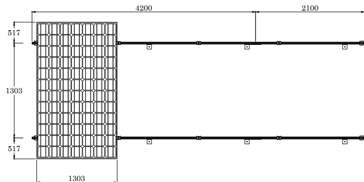
VISTA PLANTA
