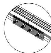
DETALLE D Empalme de Riel
