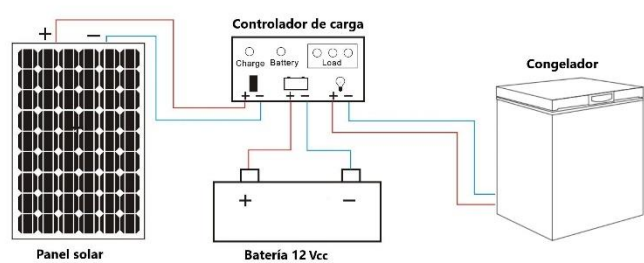
Diagrama de conexión en 12 Vcc
