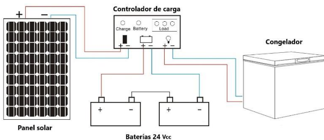
Diagrama de conexión en 24 Vcc
