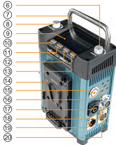
MINI MEGA-4FC / 3FC Control Box
