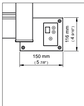
Ingombro regolatore di potenza Digital heat controller dimensions Dimensions du regulateur de puissance
