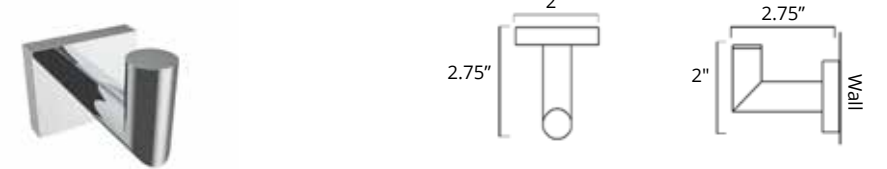
Towel Hook Crochet à serviette
