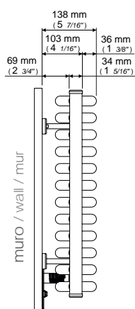
Ingombro con attacco lungo Measurements with long wall brackets Mesurations avec attache long
