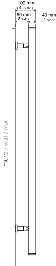
Ingombro con attacco lungo Measurements with long wall brackets Mesurations avec attache long
