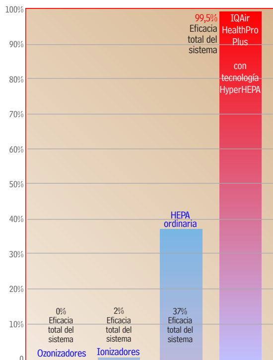
Eficacia total del sistema (retención de partículas) para tamaños de partícula: 0,01 – 1,00 micrones
