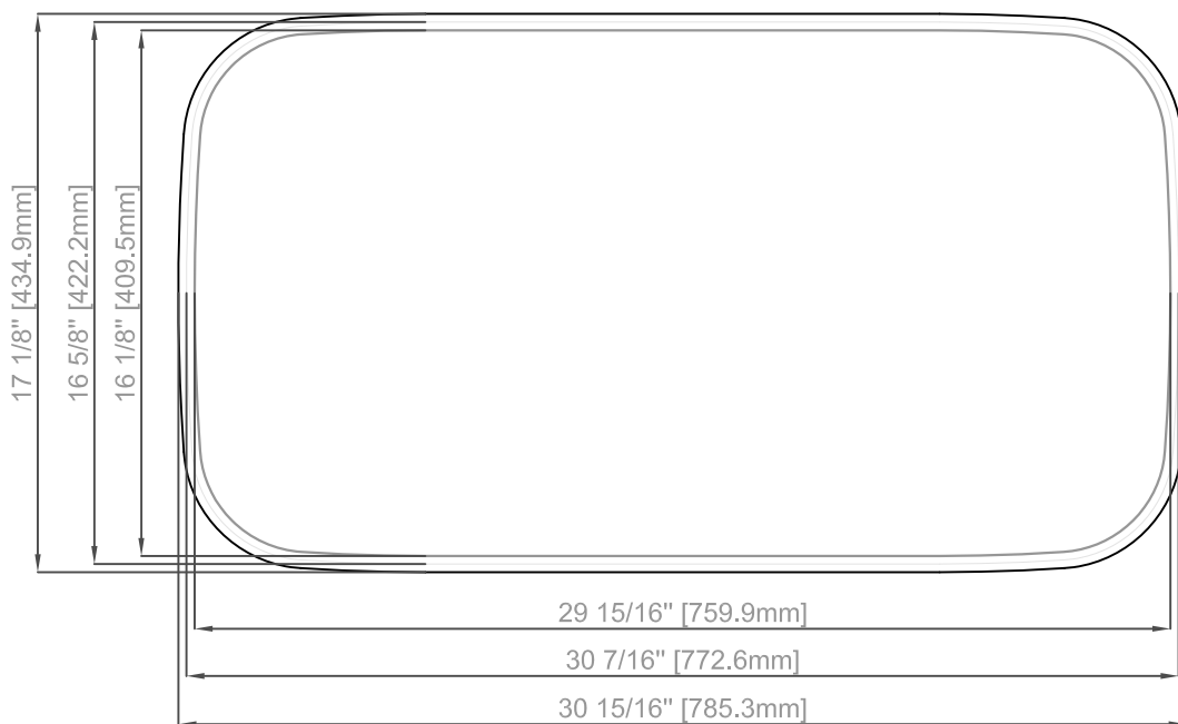
CUTOUT
