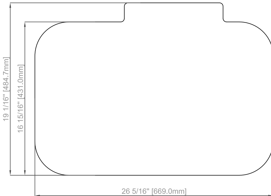
CUTOUT
