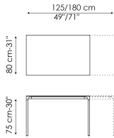
Width: 125-180cm Depth: 80cm Height: 75cm
