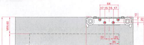
ACCESSORIES PLACEMENT (STANDARD POSITION) / POSIZIONAMENTO DEGLI ACCESSORI (POSIZIONE STANDARD)
