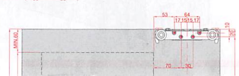
ACCESSORIES PLACEMENT (TOTAL OPENING POSITION) / POSIZIONAMENTO DEGLI ACCESSORI (POSIZIONE APERTURA TOTALE)
