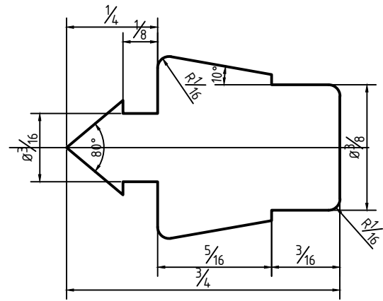
B-B (5:1)
