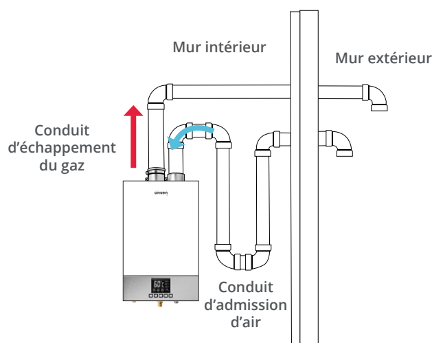
Figure 2: Ventilation directe (air de combustion provenant de l'extérieur)
