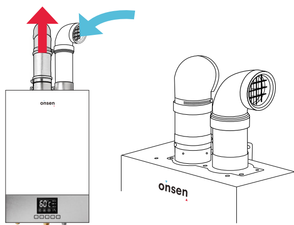
Figure 1: Ventilation indirecte (air de combustion provenant de la pièce)
