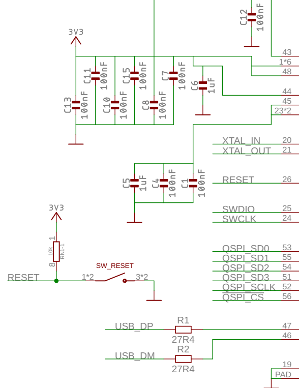
RP2040 MCU
