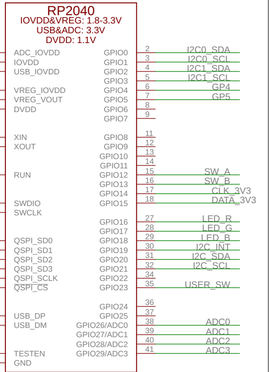
MCU1
