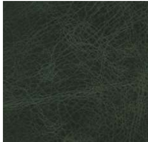
Thyme
