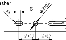
Mounting hole 安装孔位
