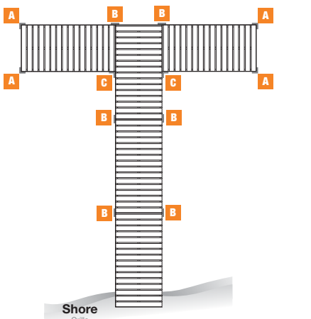
Shore Orilla 5 Dock Kits Kits de 5 tramos de muelles
