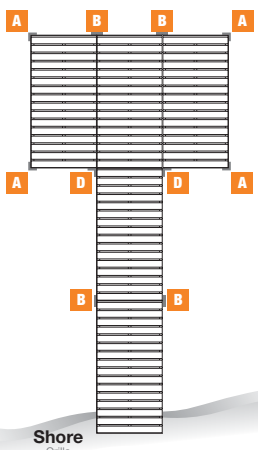
Shore Orilla 5 Dock Kits Kits de 5 tramos de muelles
