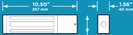
1216-080 / 1216-081 DKGL-S12-1 / DKGL-S12-1L
