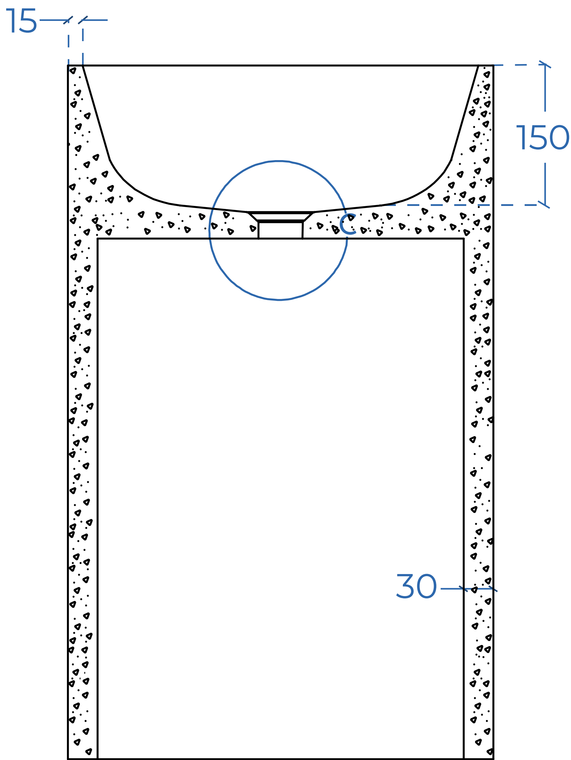
Section A-A
