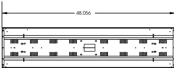
48L - 48"L x 11.385"W
