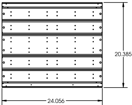
22L - 24.056"L x 20.385"W
