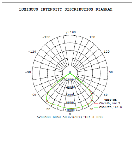
150W 4K 110° Optic
