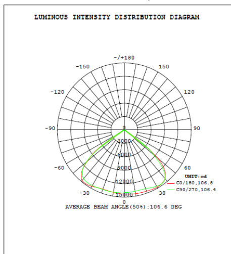
240W 4K 110° Optic
