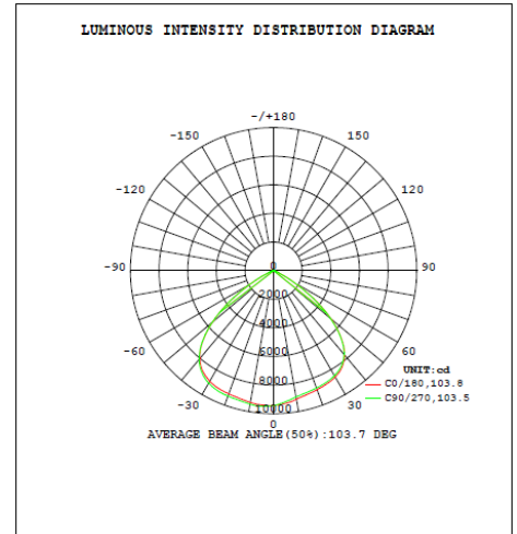
150W 4K 110° Optic
