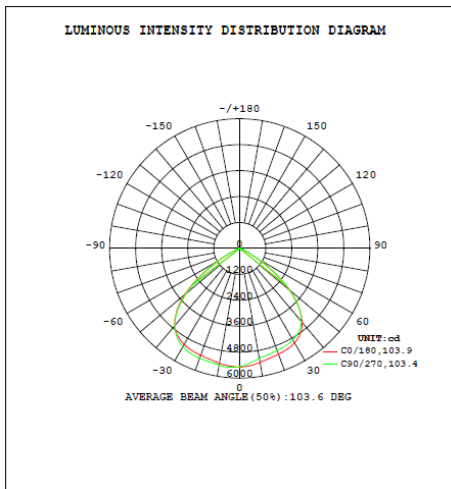
80W 4K 110° Optic
