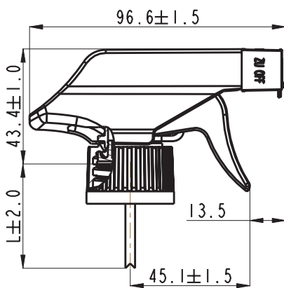
Section A-A Scale 0.500
