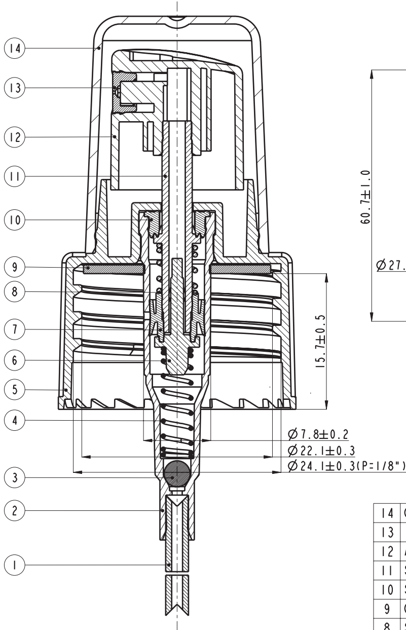
Section A-A
