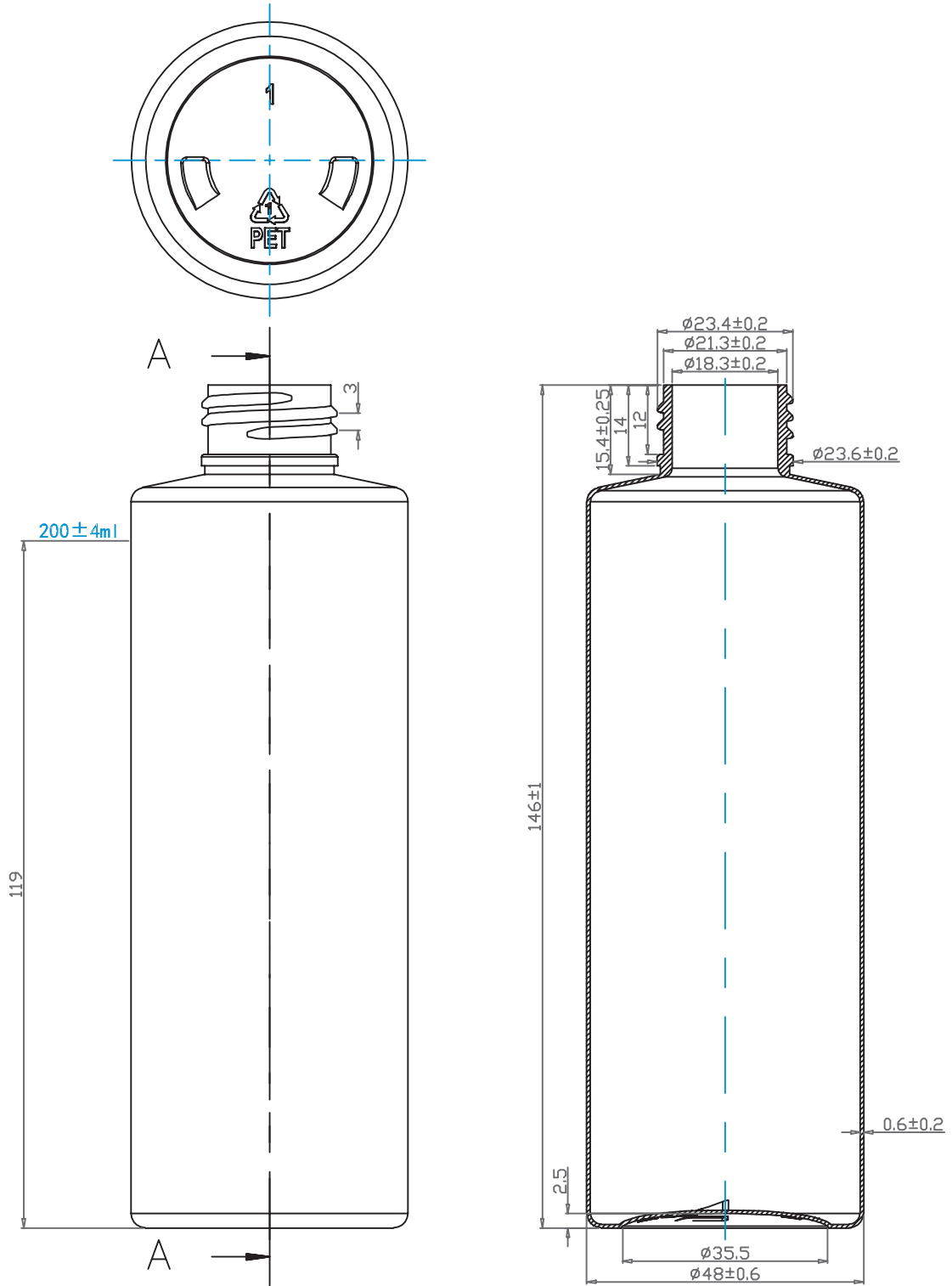
SECTION A-A
