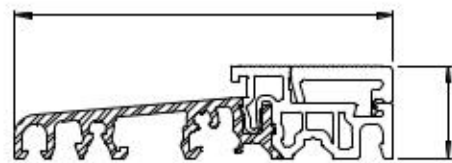
216325 dorpel
