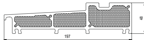
279110 dorpel
