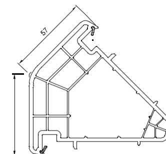
416 240 Hoekkoppeling 135°
