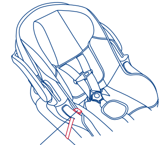
Short clip Gancho corto Agrafe courte Fig. 11c
