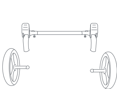
Rear Axle and (2) Wheels Eje trasero y (2) Ruedas Essieu arrière et (2) Roues
