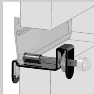
binnendraaiende brievenbus
