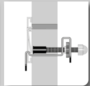
binnendraaiende brievenbus
