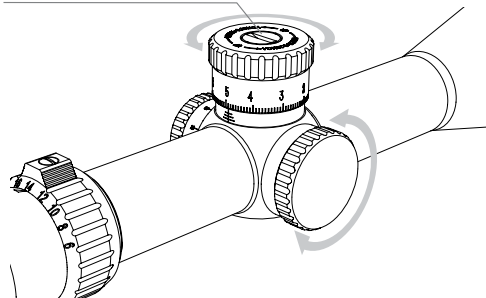
Vis de centre de la molette de hauteur (Capuchon tourelle de dérive)
